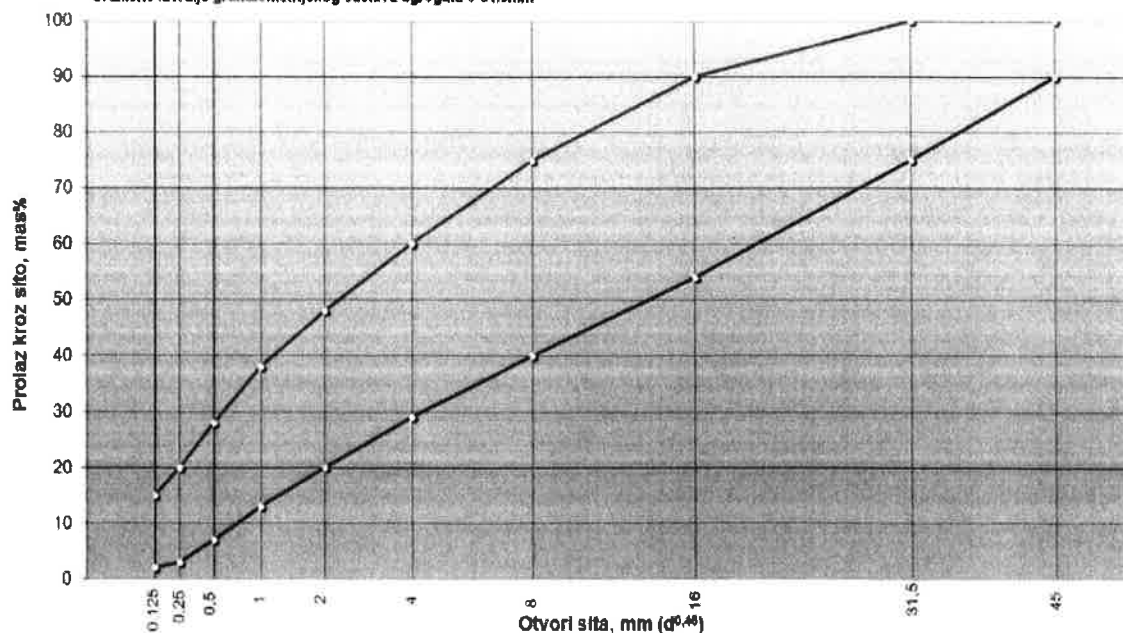
Dijagram 1. Anvelope granulometrijskih krivulja za zaštitni sloj
