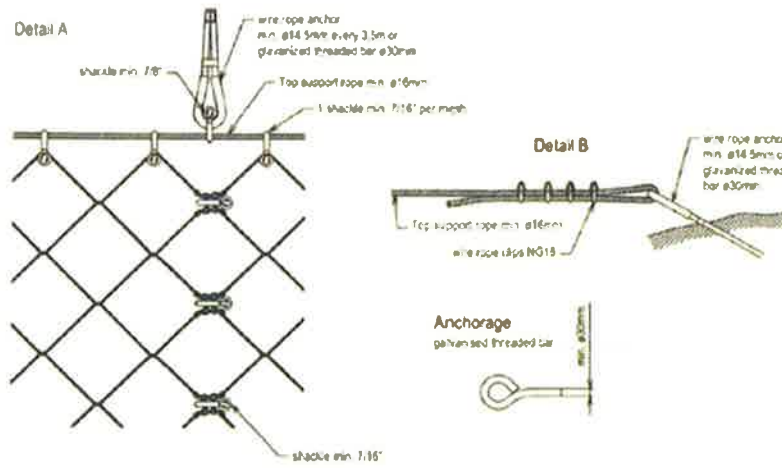
1. Mreža – varijanta zaštite TIP2 (detalji)
