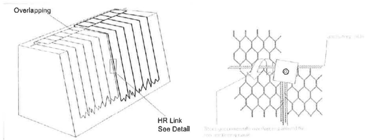
4. Detalj preklapanja mreža – DETALJ "A"
