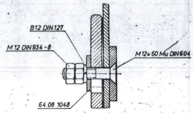
Schnitt L-M M 1:1
